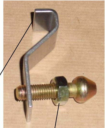
3b Kugelbolzen mit Mutter
